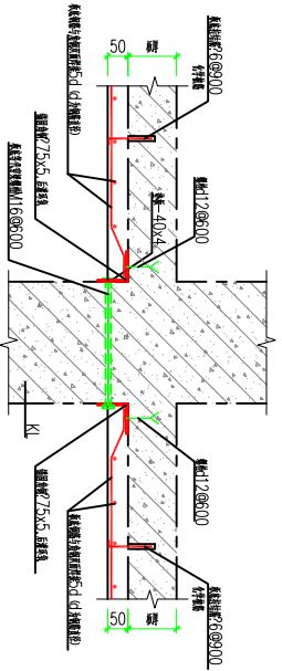
2-2 断面 1:10
