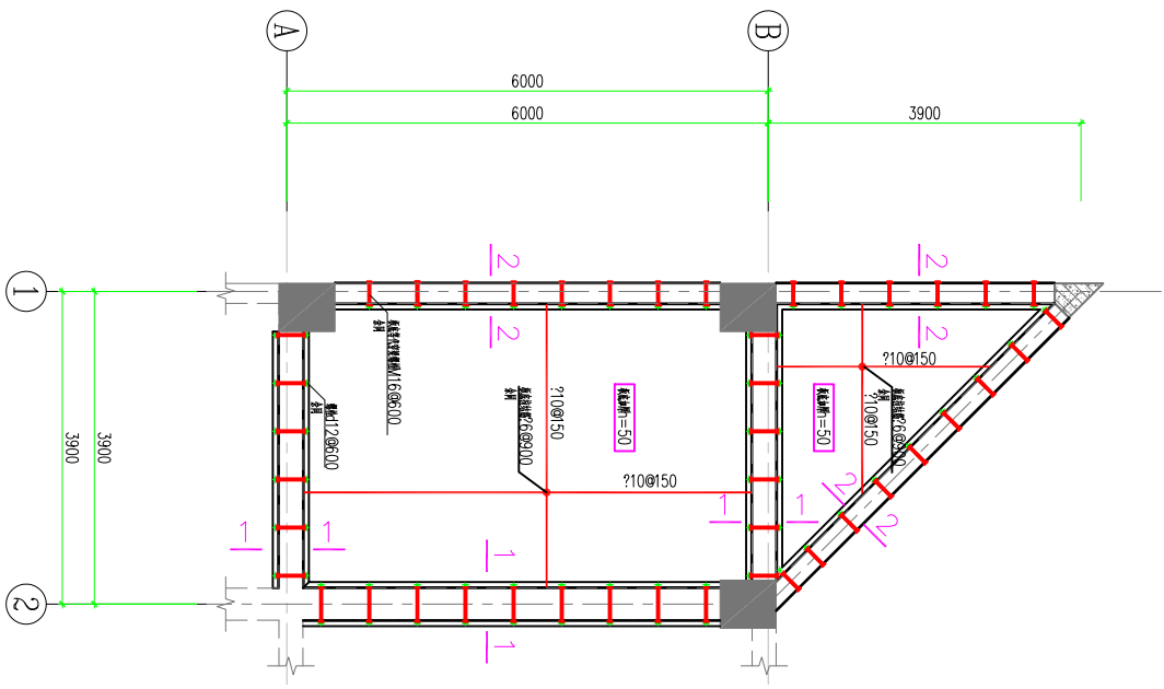
结构平面布置 1:50
